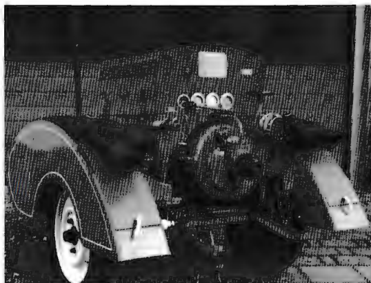
franz. Motorpumpe TS 5/8 Fabrikat: Maheu - Labrosse; Baujahr 1948; Antrieb: 4 Takt Peugeot 202; Leistung 500 l/min bei 8 bar; Gew. ca. 300 kg Heutiger Standort: Feuerwehrmuseum Hermeskeil
